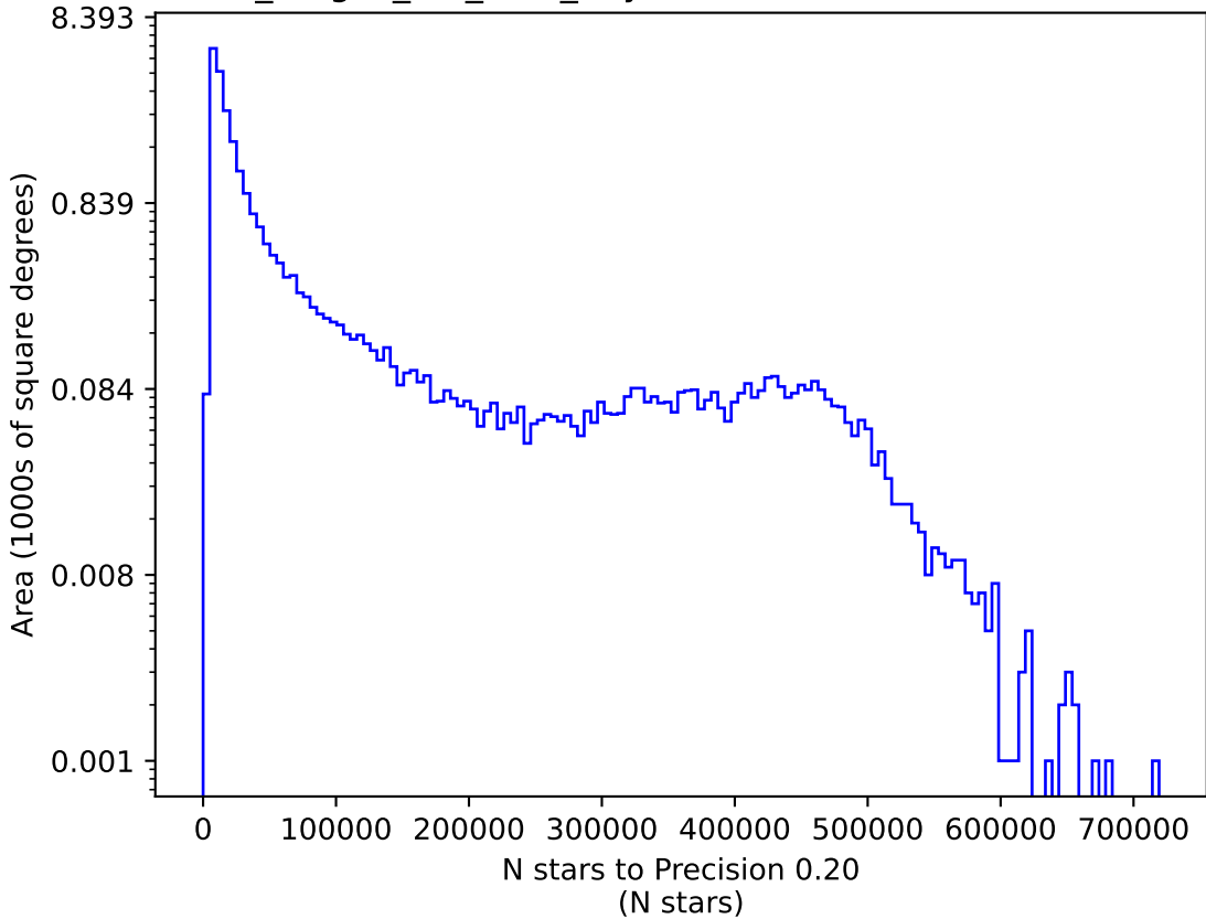
no_magell_roll_v3.4_10yrs i: N stars to Precision 0.20
