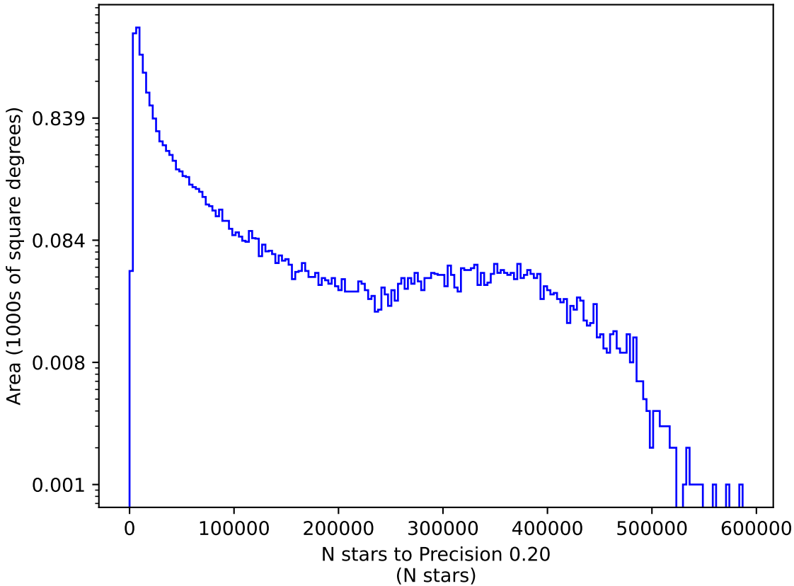
no_magell_roll_v3.4_10yrs g: N stars to Precision 0.20
