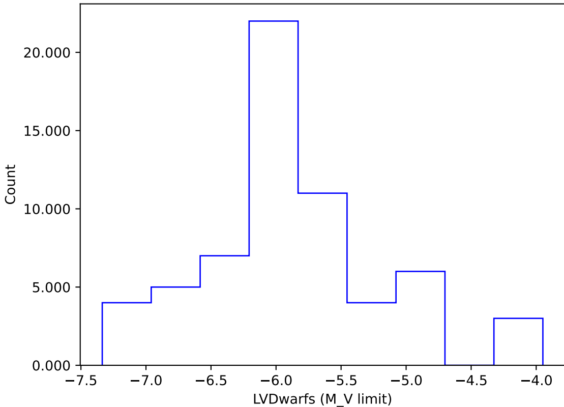
no_magell_roll_v3.4_10yrs gi: LVDwarfs
