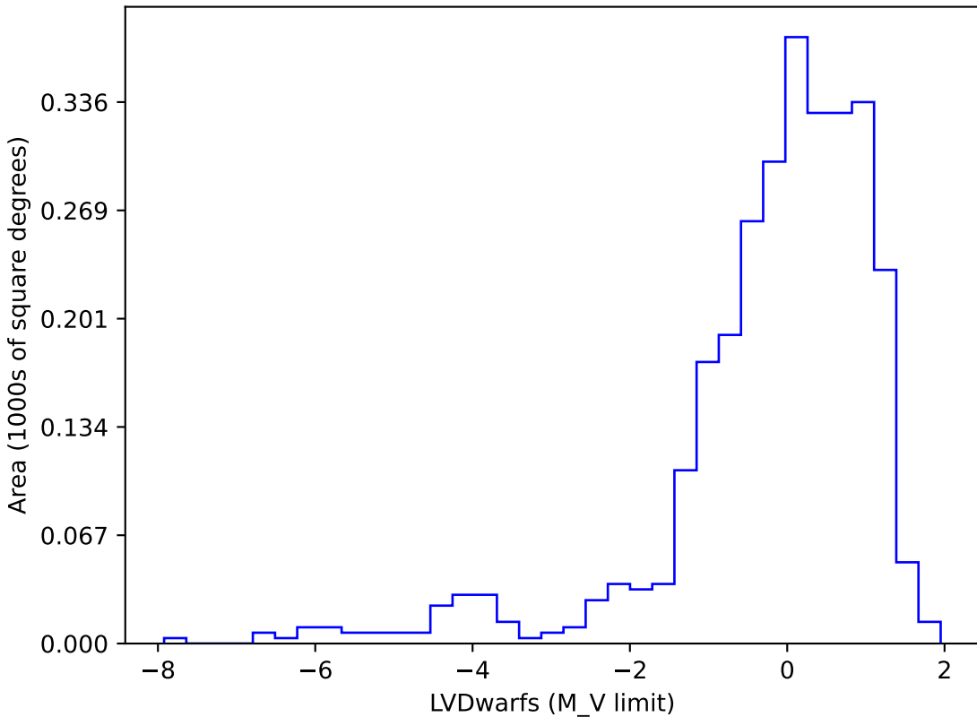
no_magell_roll_v3.4_10yrs gi SCP: LVDwarfs
