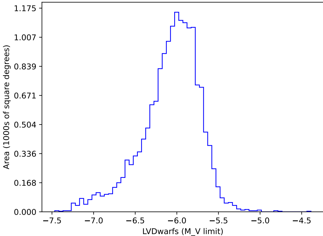
no_magell_roll_v3.4_10yrs gi: LVDwarfs
