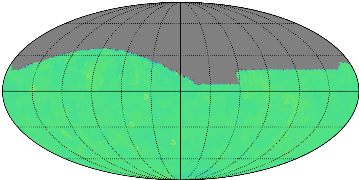
no_magell_roll_v3.4_10yrs z: Kuiper rotTelPos
