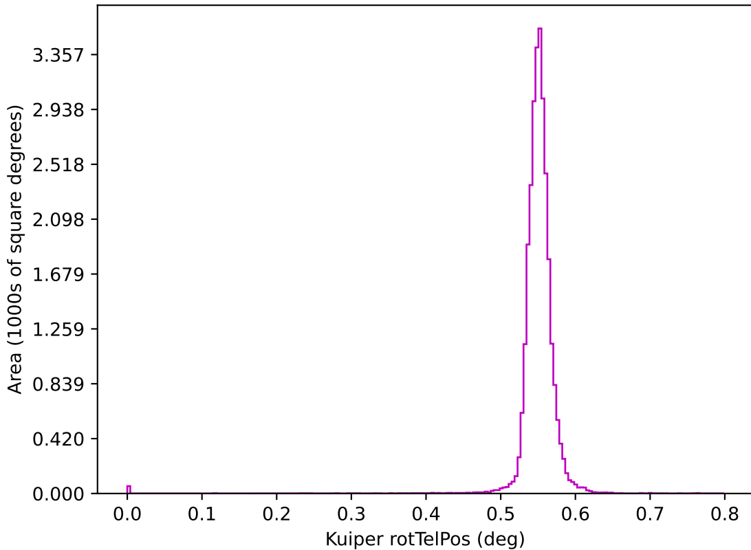
no_magell_roll_v3.4_10yrs z: Kuiper rotTelPos
