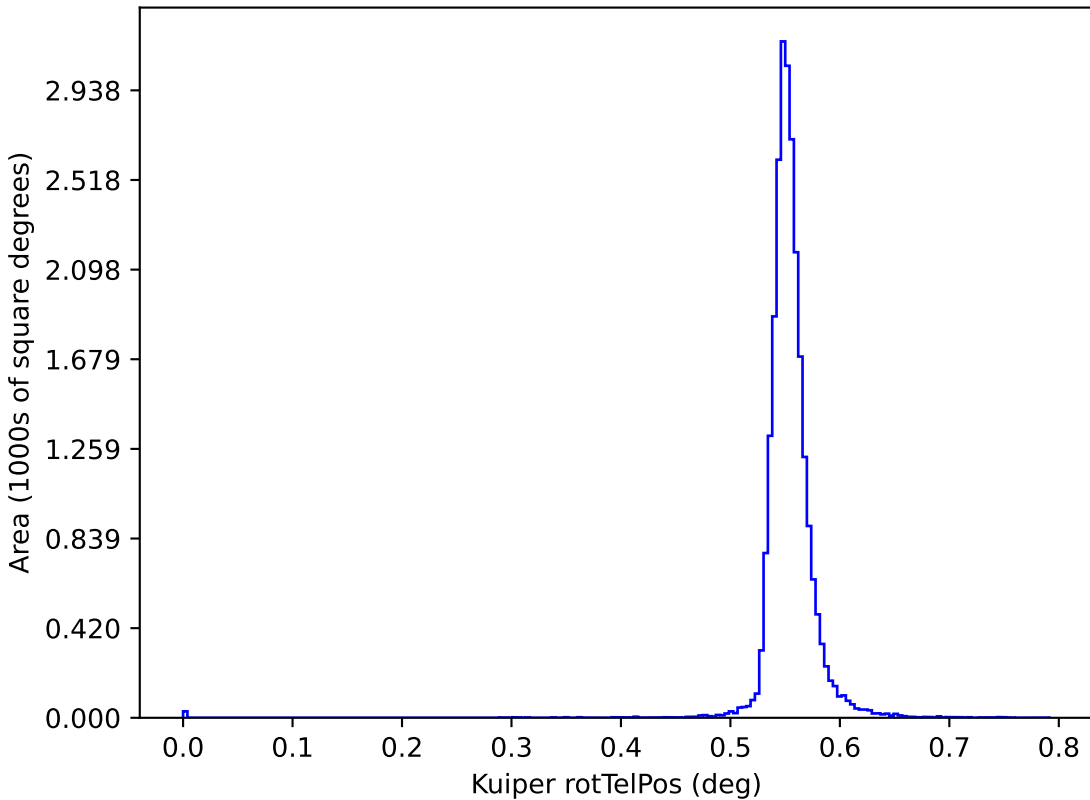
no_magell_roll_v3.4_10yrs y: Kuiper rotTelPos
