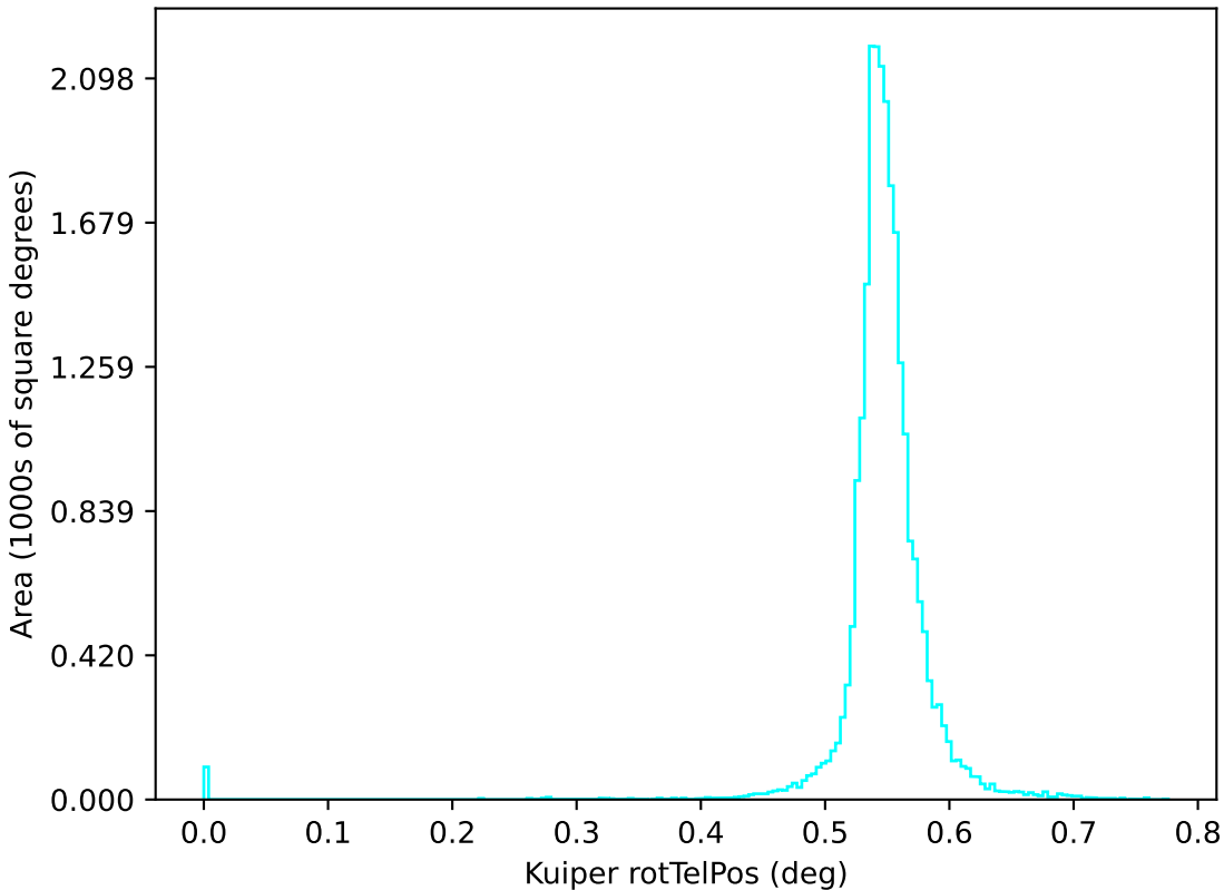
no_magell_roll_v3.4_10yrs u: Kuiper rotTelPos
