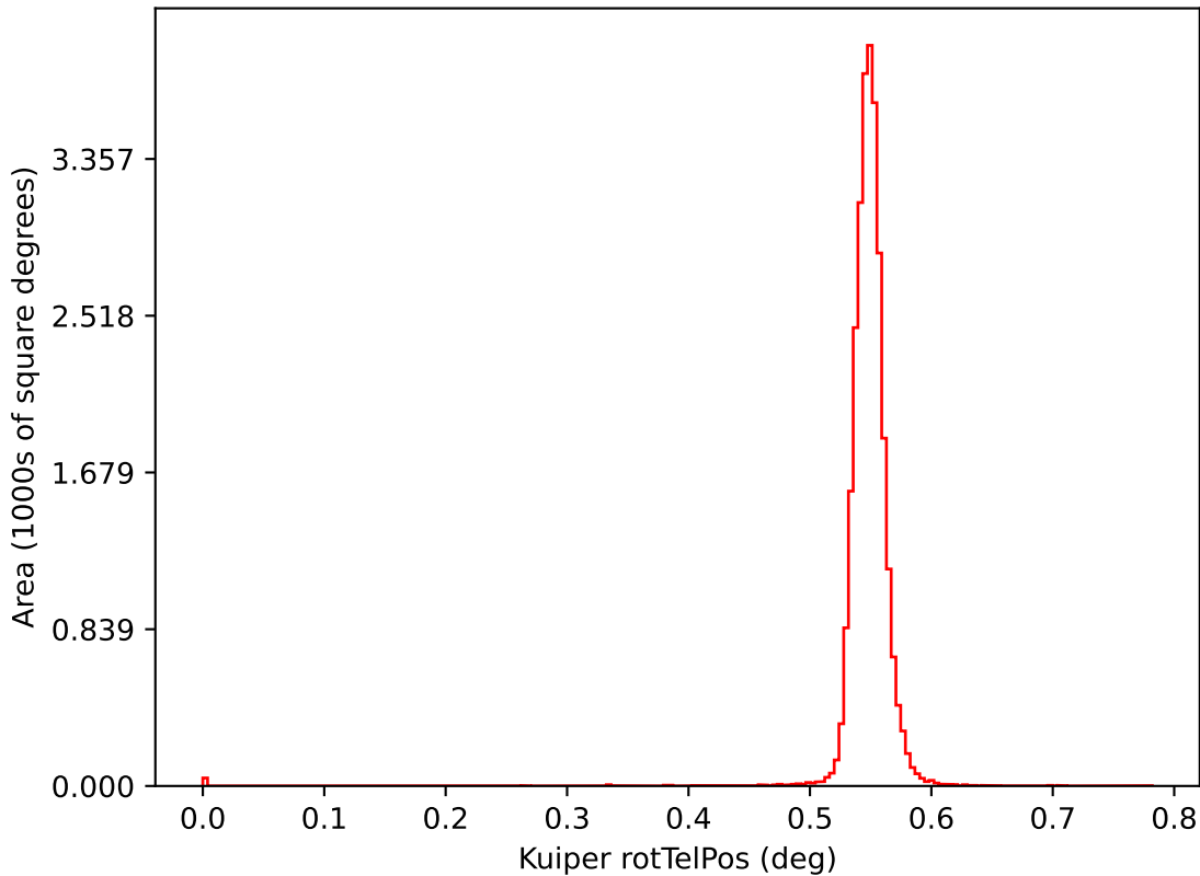
no_magell_roll_v3.4_10yrs i: Kuiper rotTelPos
