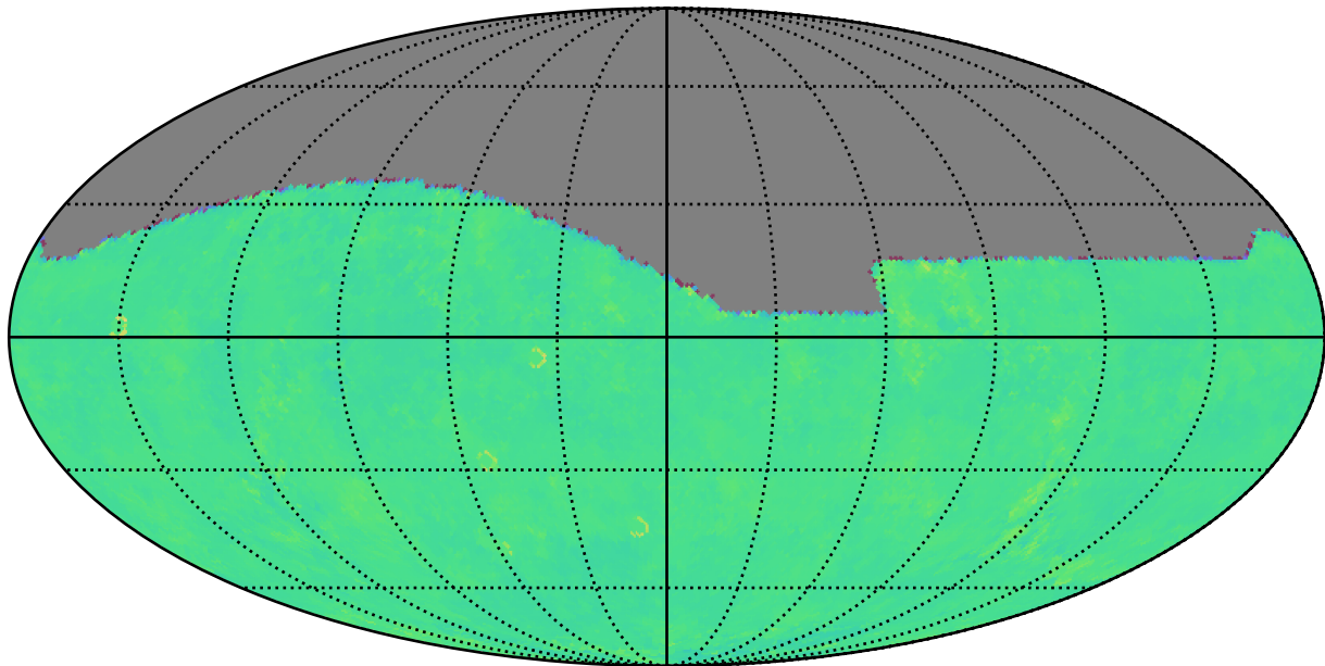
no_magell_roll_v3.4_10yrs g: Kuiper rotTelPos
