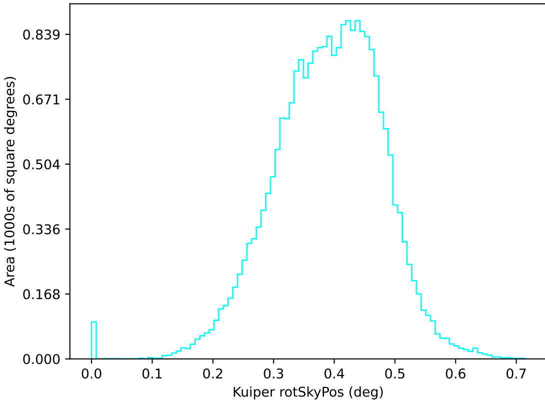
no_magell_roll_v3.4_10yrs u: Kuiper rotSkyPos
