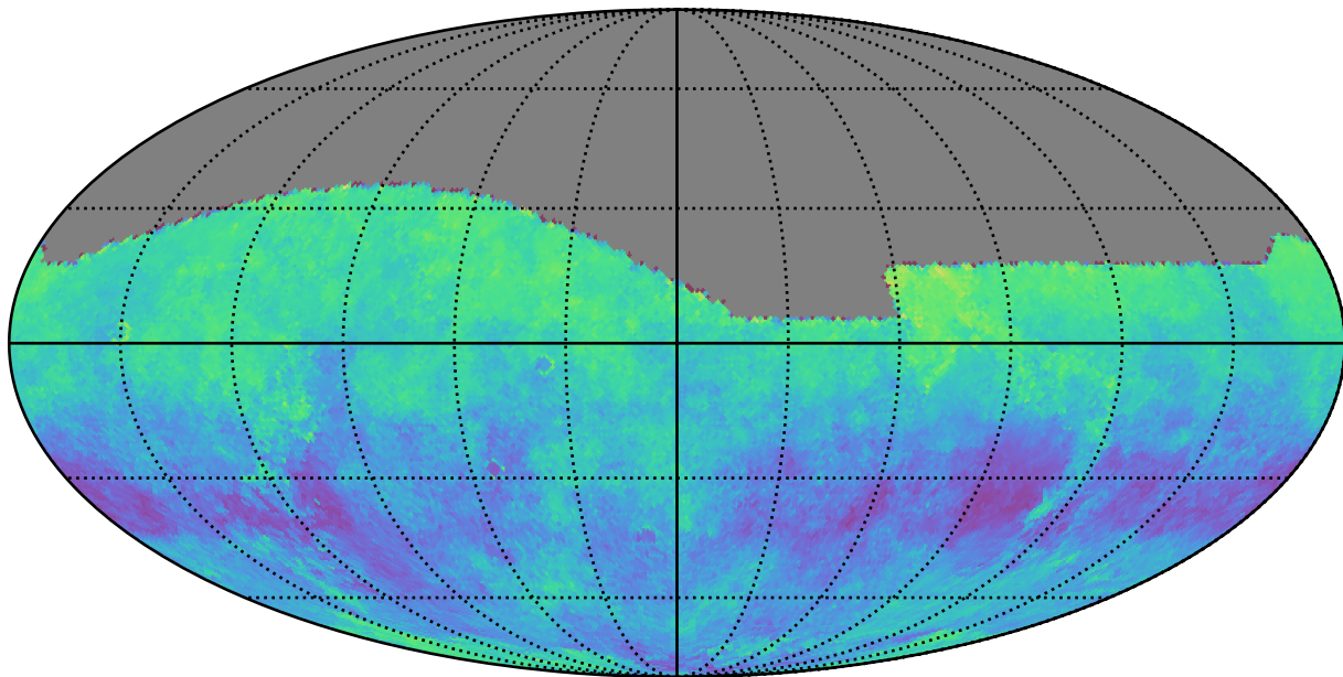
no_magell_roll_v3.4_10yrs g: Kuiper rotSkyPos
