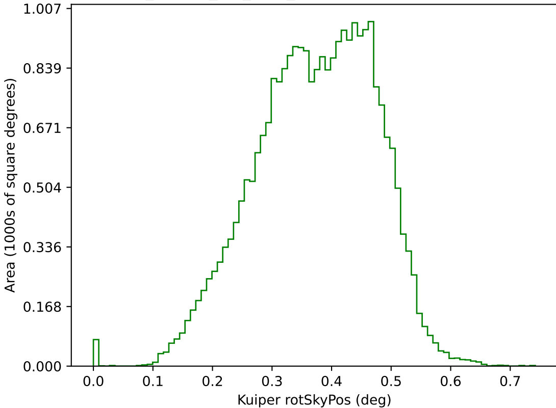
no_magell_roll_v3.4_10yrs g: Kuiper rotSkyPos
