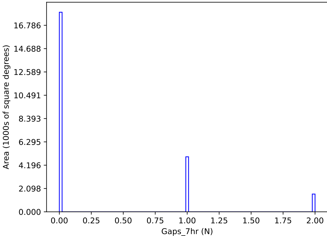
no_magell_roll_v3.4_10yrs y band: Gaps_7hr
