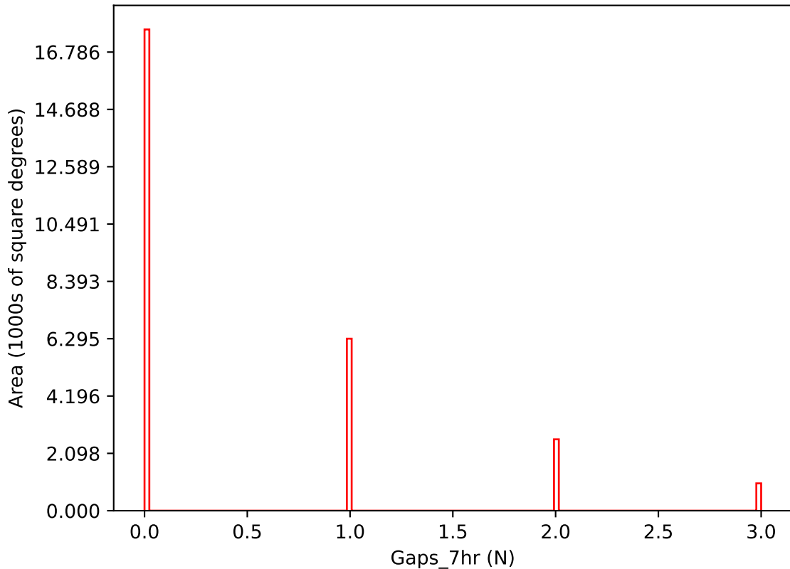
no_magell_roll_v3.4_10yrs i band: Gaps_7hr
