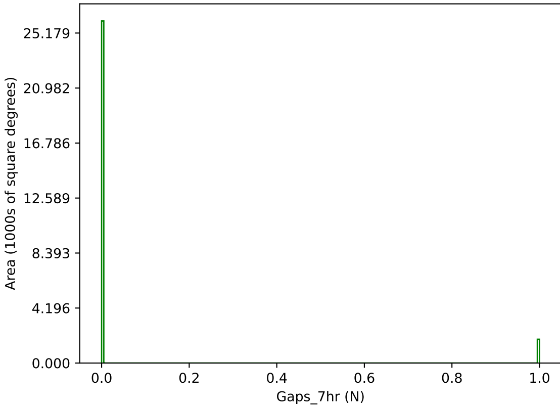
no_magell_roll_v3.4_10yrs g band: Gaps_7hr
