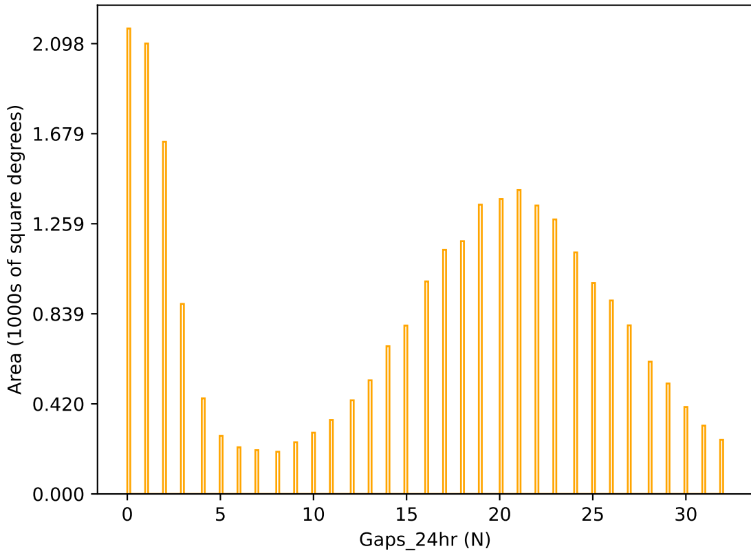
no_magell_roll_v3.4_10yrs r band: Gaps_24hr
