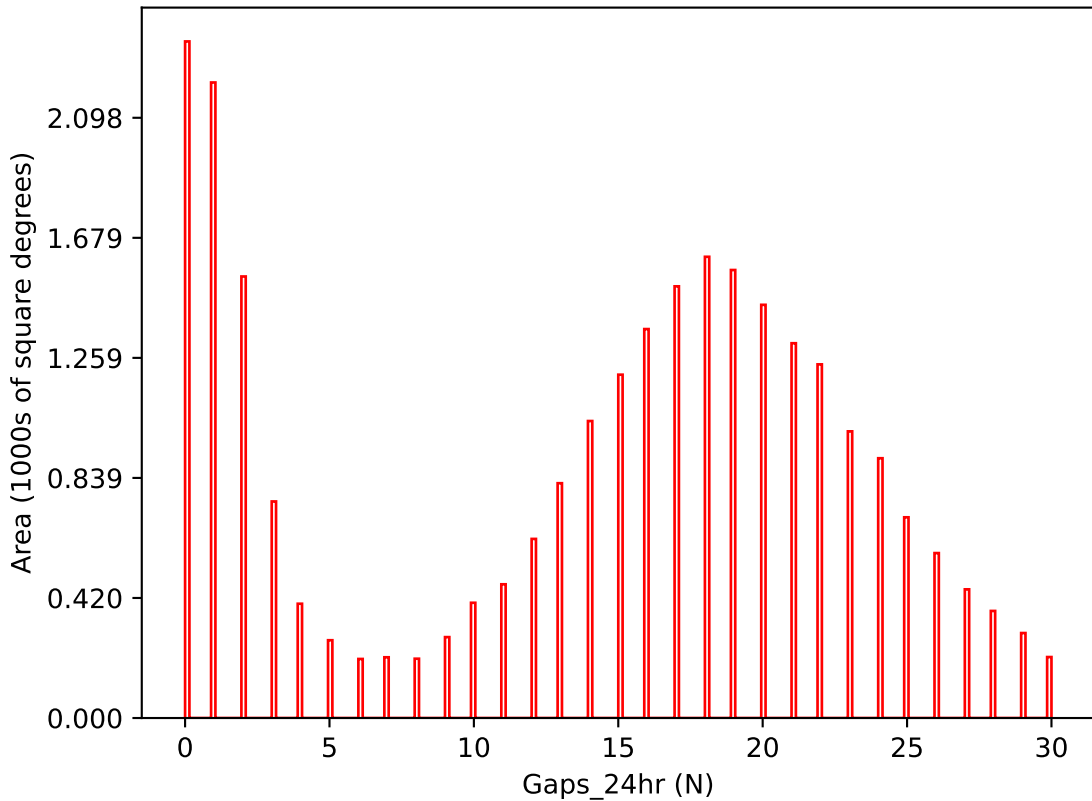
no_magell_roll_v3.4_10yrs i band: Gaps_24hr
