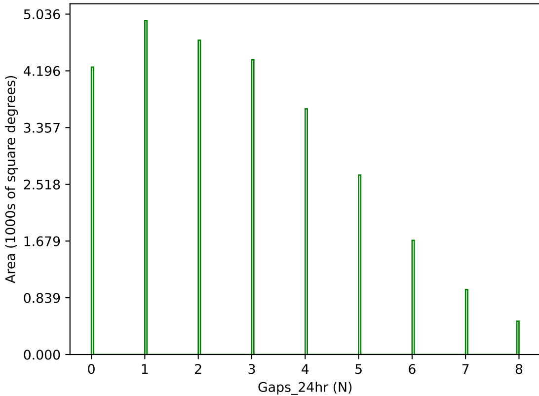
no_magell_roll_v3.4_10yrs g band: Gaps_24hr
