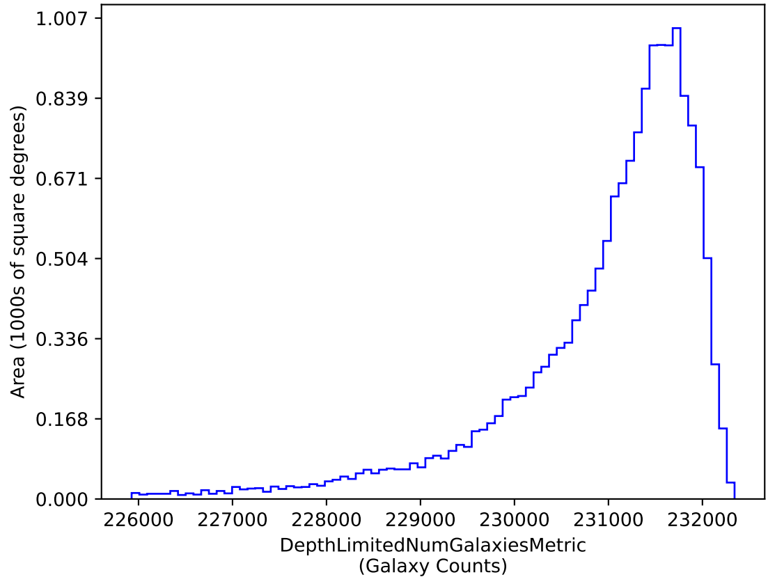
no_magell_roll_v3.4_10yrs i band galaxies non-DD: DepthLimitedNumGalaxiesMetric
