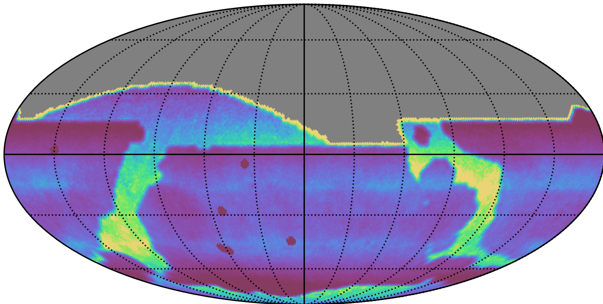
no_magell_roll_v3.4_10yrs : DCRprecision
