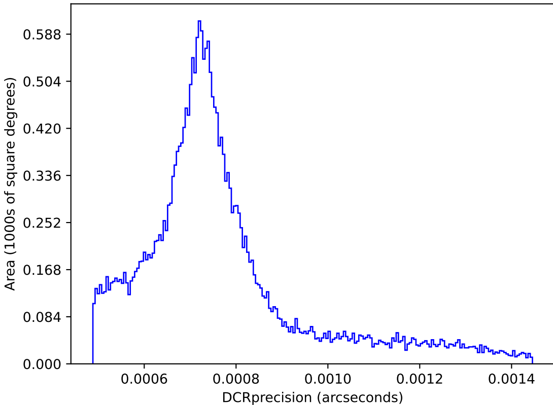
no_magell_roll_v3.4_10yrs : DCRprecision
