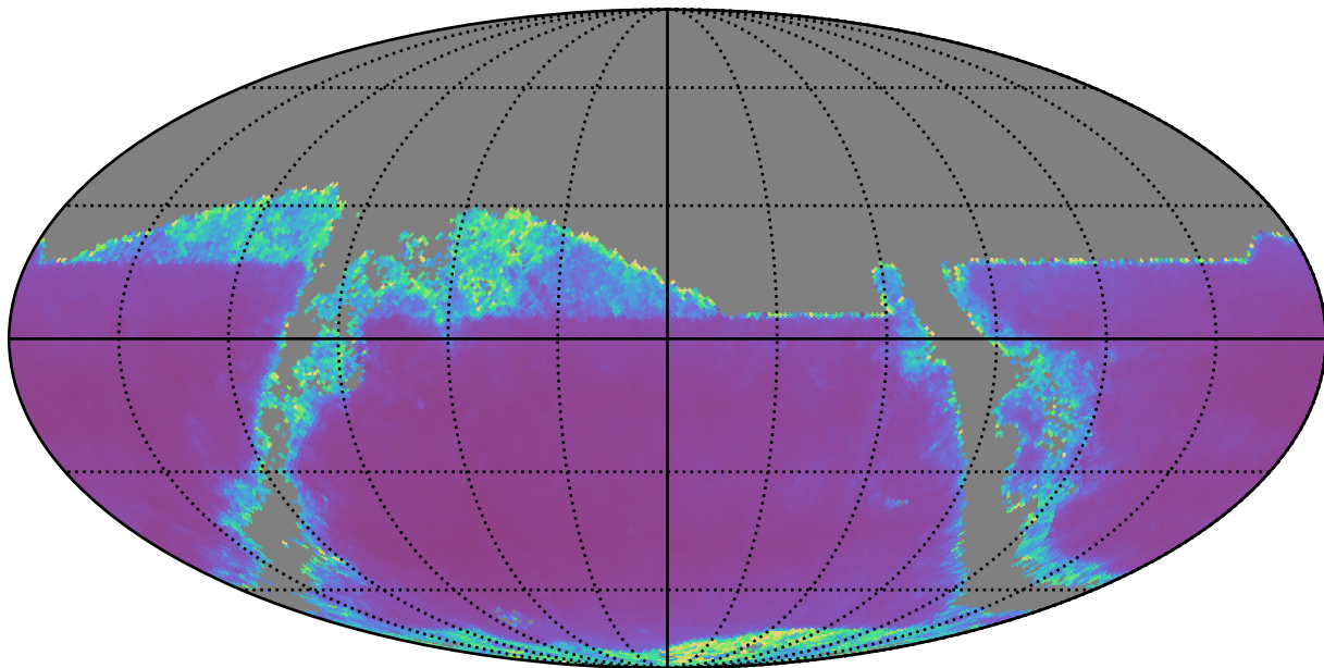
no_magell_roll_v3.4_10yrs z band: AGN SF_uncert
