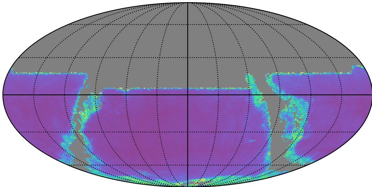
no_magell_roll_v3.4_10yrs y band: AGN SF_uncert
