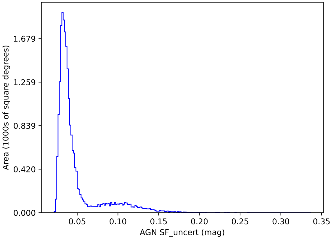
no_magell_roll_v3.4_10yrs y band: AGN SF_uncert
