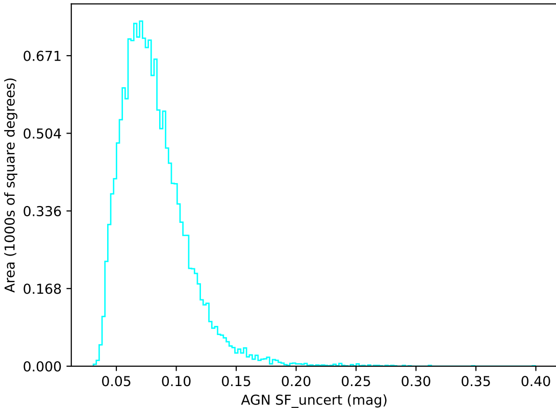
no_magell_roll_v3.4_10yrs u band: AGN SF_uncert
