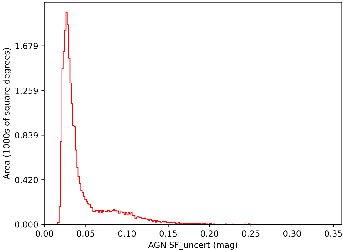
no_magell_roll_v3.4_10yrs i band: AGN SF_uncert
