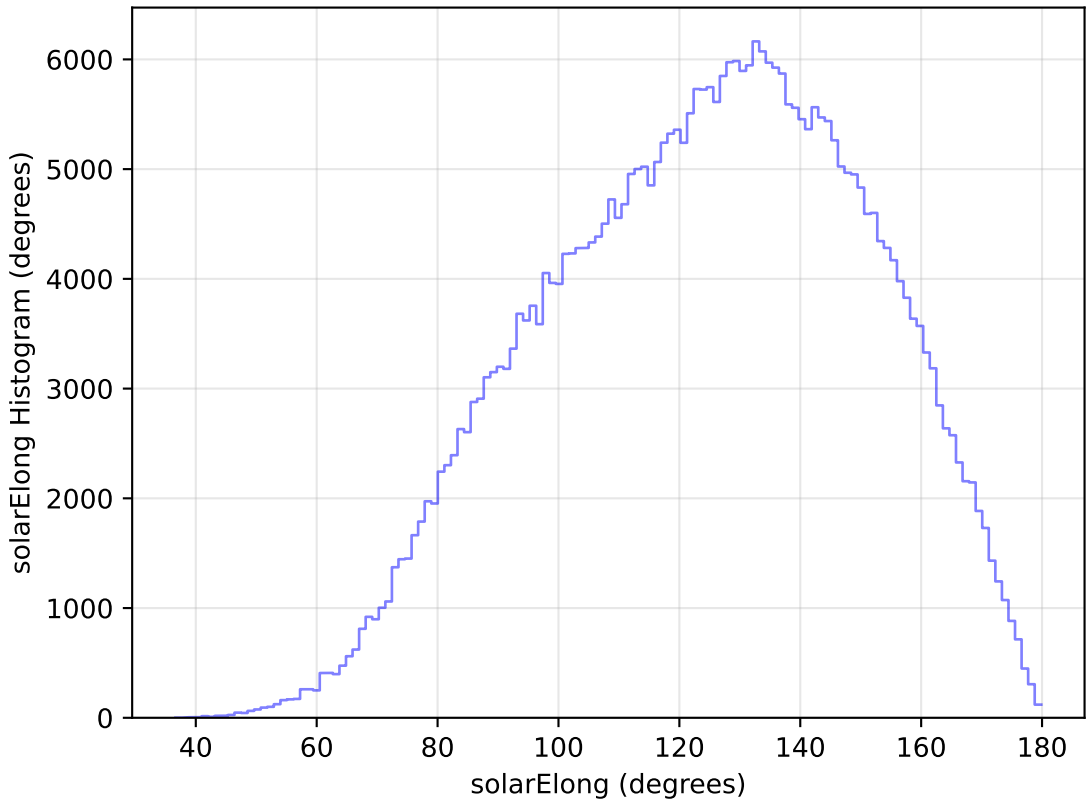
no_magell_roll_v3.4_10yrs WFD y band: solarElong Histogram
