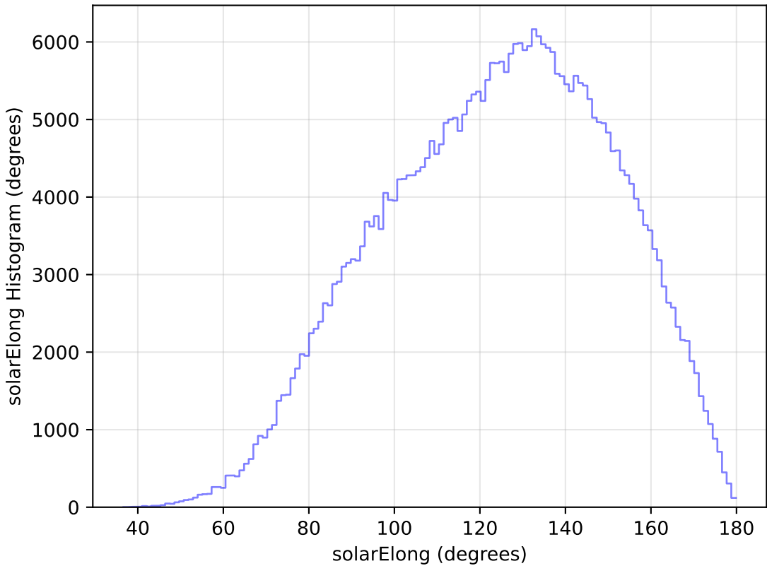
no_magell_roll_v3.4_10yrs All sky y band: solarElong Histogram
