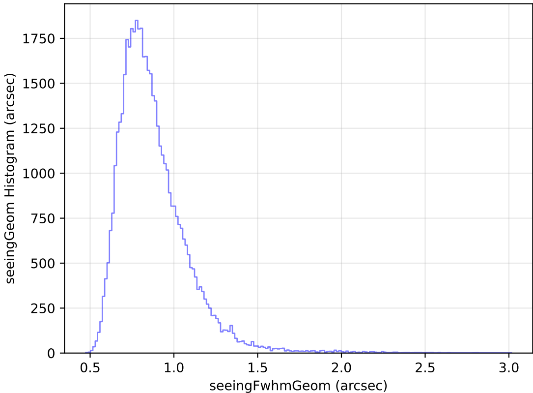
no_magell_roll_v3.4_10yrs Yr 1 y band: seeingGeom Histogram
