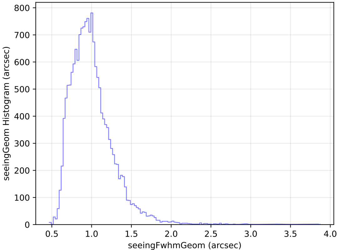
no_magell_roll_v3.4_10yrs Yr 1 u band: seeingGeom Histogram
