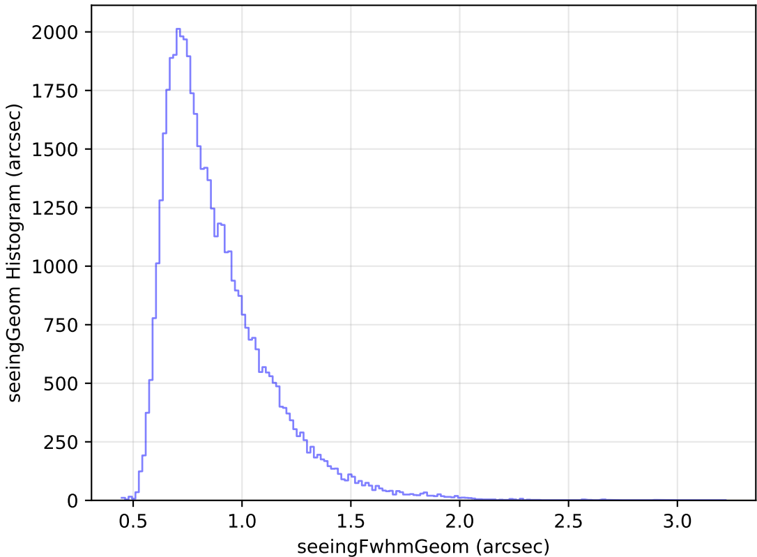
no_magell_roll_v3.4_10yrs Yr 1 r band: seeingGeom Histogram
