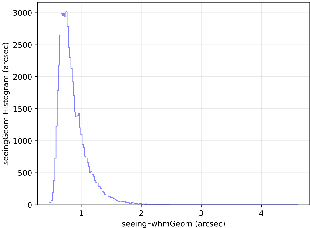
no_magell_roll_v3.4_10yrs Yr 1 i band: seeingGeom Histogram
