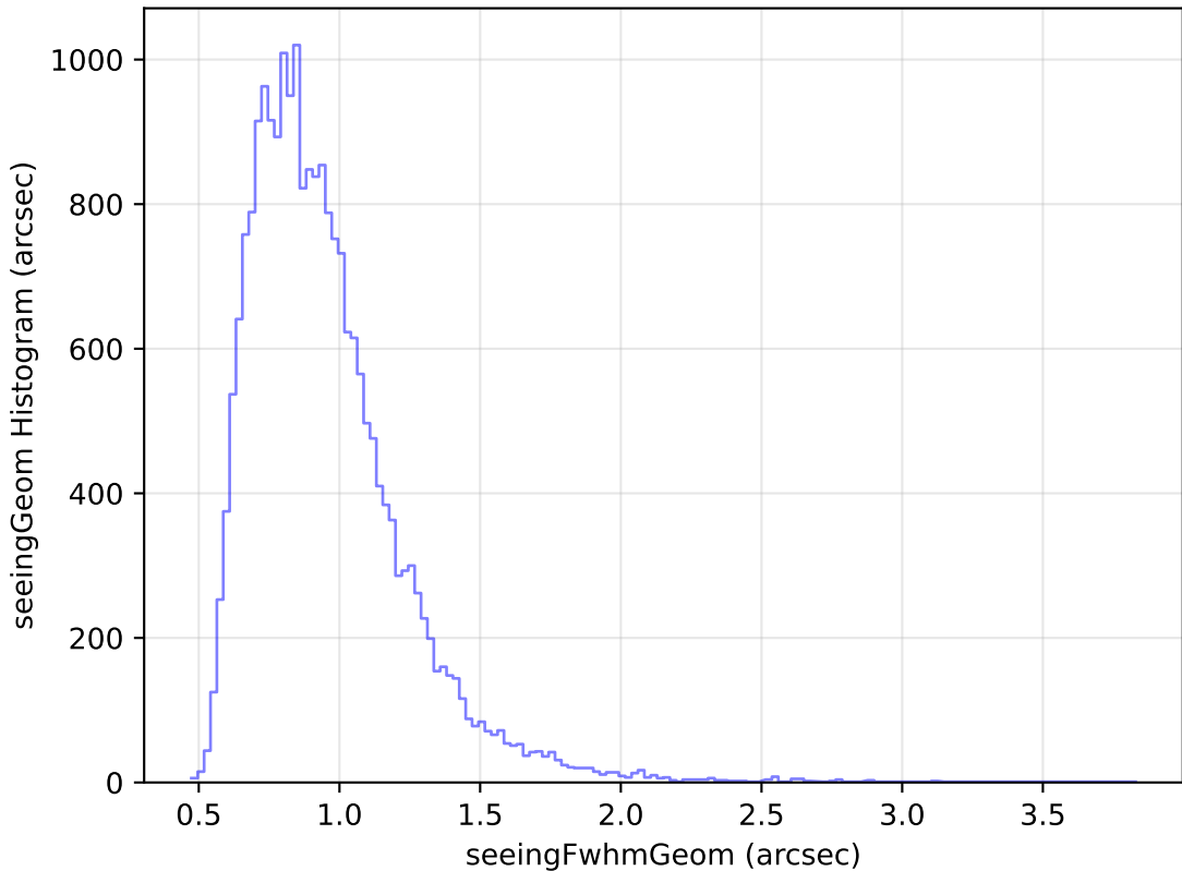
no_magell_roll_v3.4_10yrs Yr 1 g band: seeingGeom Histogram
