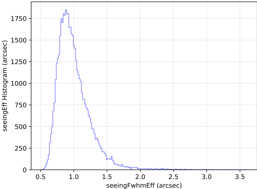
no_magell_roll_v3.4_10yrs Yr 1 y band: seeingEff Histogram
