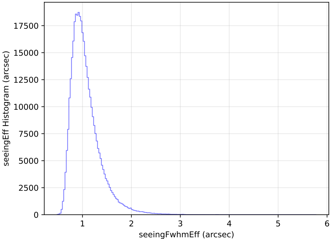
no_magell_roll_v3.4_10yrs WFD y band: seeingEff Histogram
