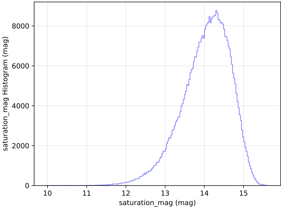
no_magell_roll_v3.4_10yrs WFD z band: saturation_mag Histogram
