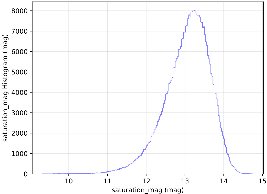
no_magell_roll_v3.4_10yrs WFD y band: saturation_mag Histogram
