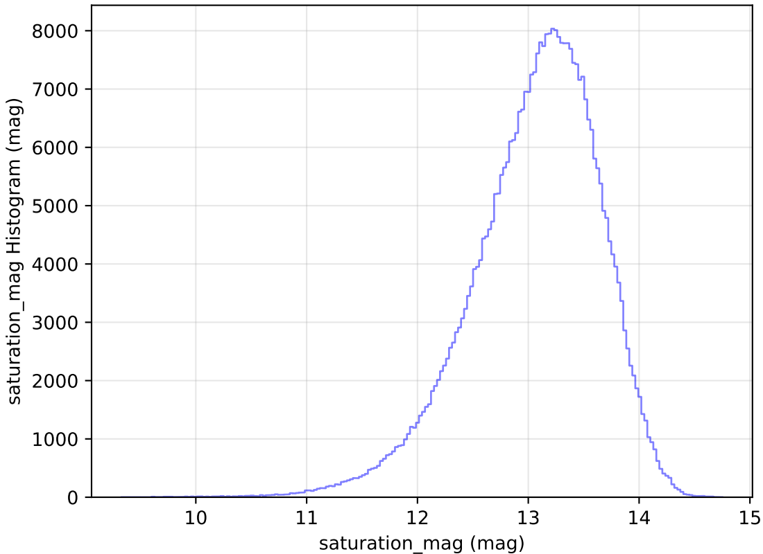
no_magell_roll_v3.4_10yrs All sky y band: saturation_mag Histogram
