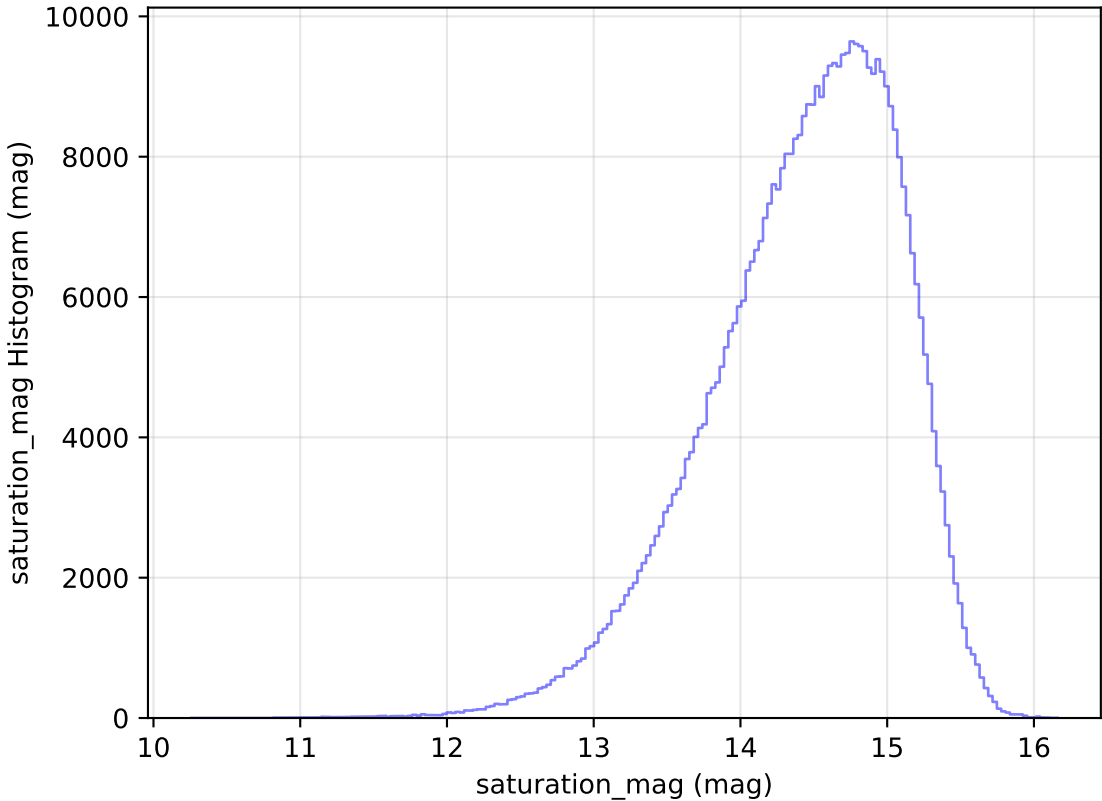
no_magell_roll_v3.4_10yrs All sky i band: saturation_mag Histogram
