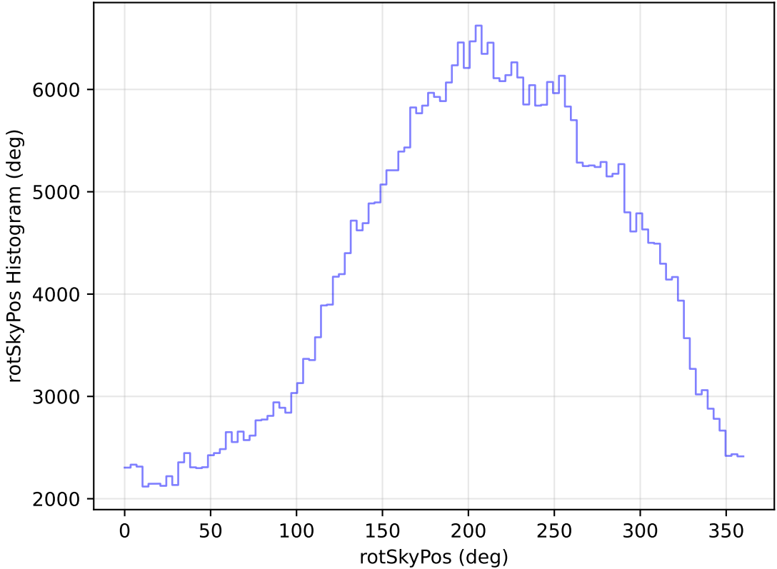
no_magell_roll_v3.4_10yrs WFD z band: rotSkyPos Histogram
