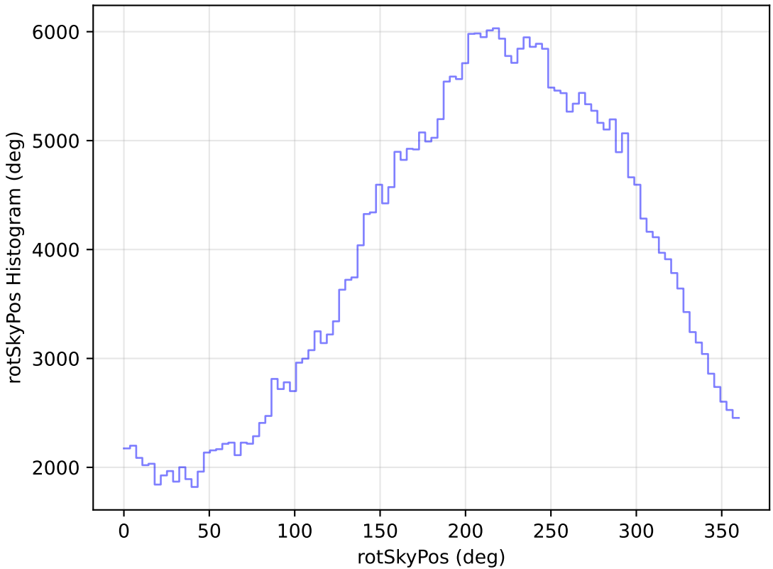
no_magell_roll_v3.4_10yrs WFD y band: rotSkyPos Histogram
