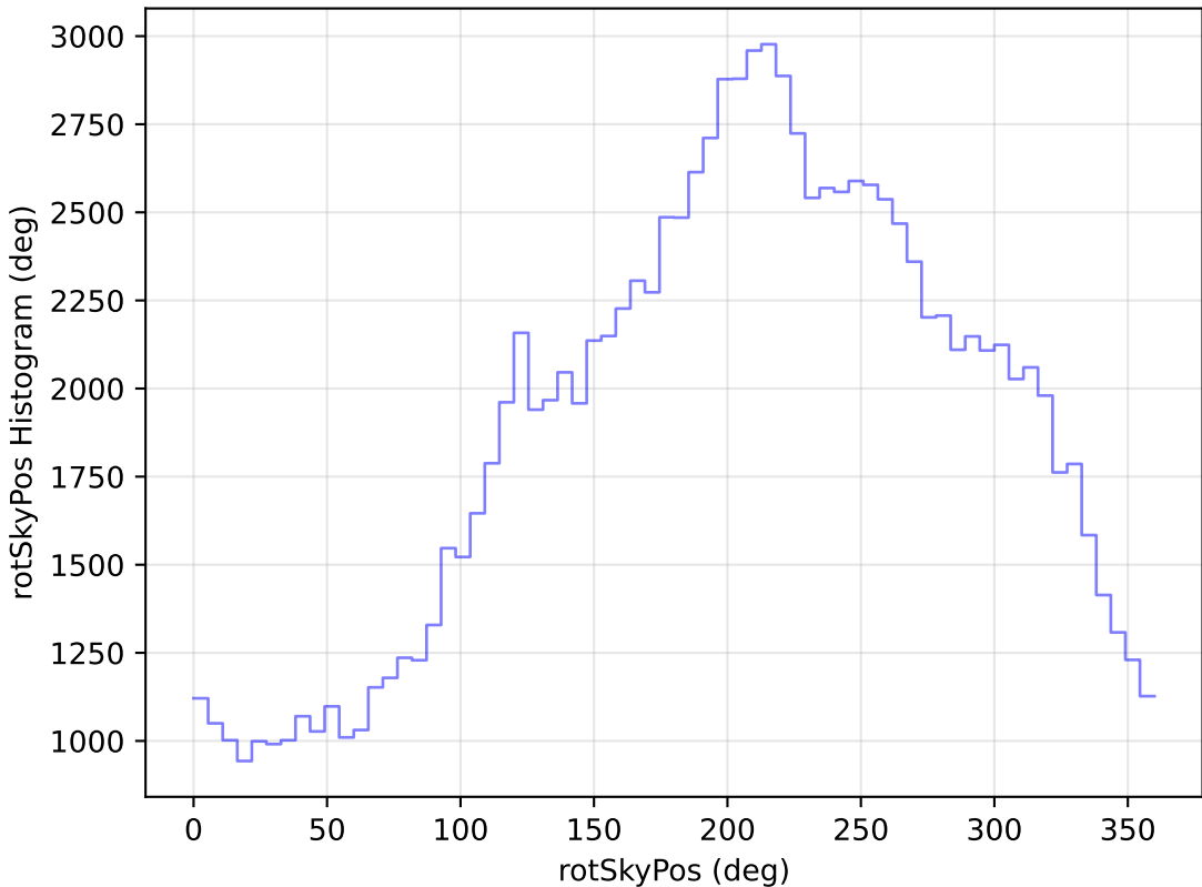
no_magell_roll_v3.4_10yrs WFD u band: rotSkyPos Histogram
