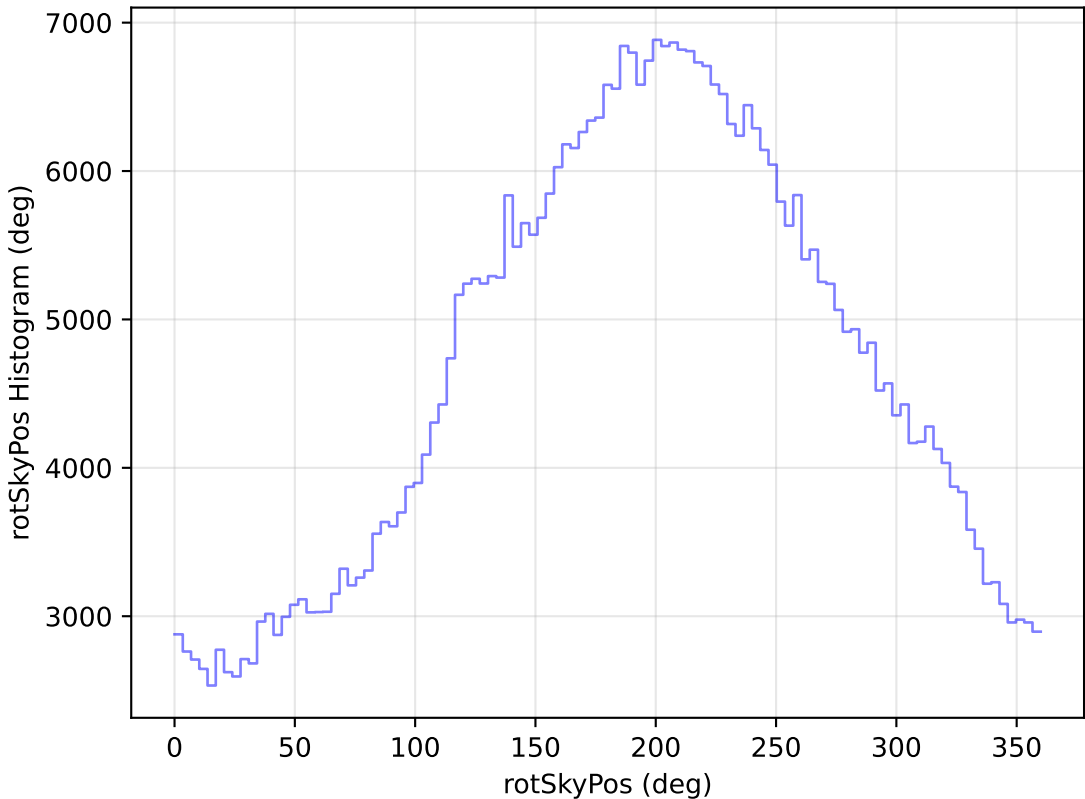
no_magell_roll_v3.4_10yrs WFD r band: rotSkyPos Histogram
