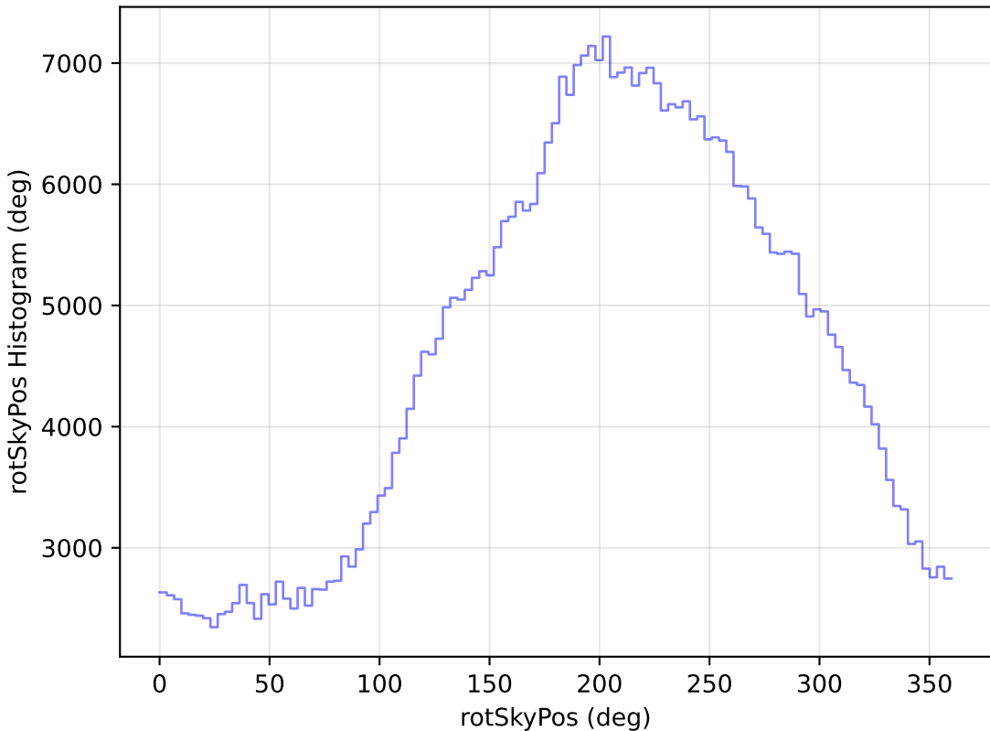
no_magell_roll_v3.4_10yrs WFD i band: rotSkyPos Histogram
