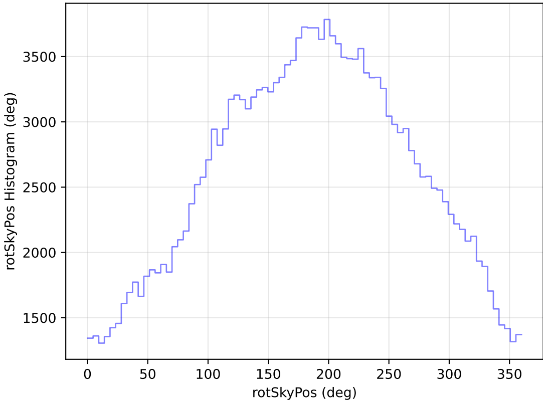
no_magell_roll_v3.4_10yrs WFD g band: rotSkyPos Histogram
