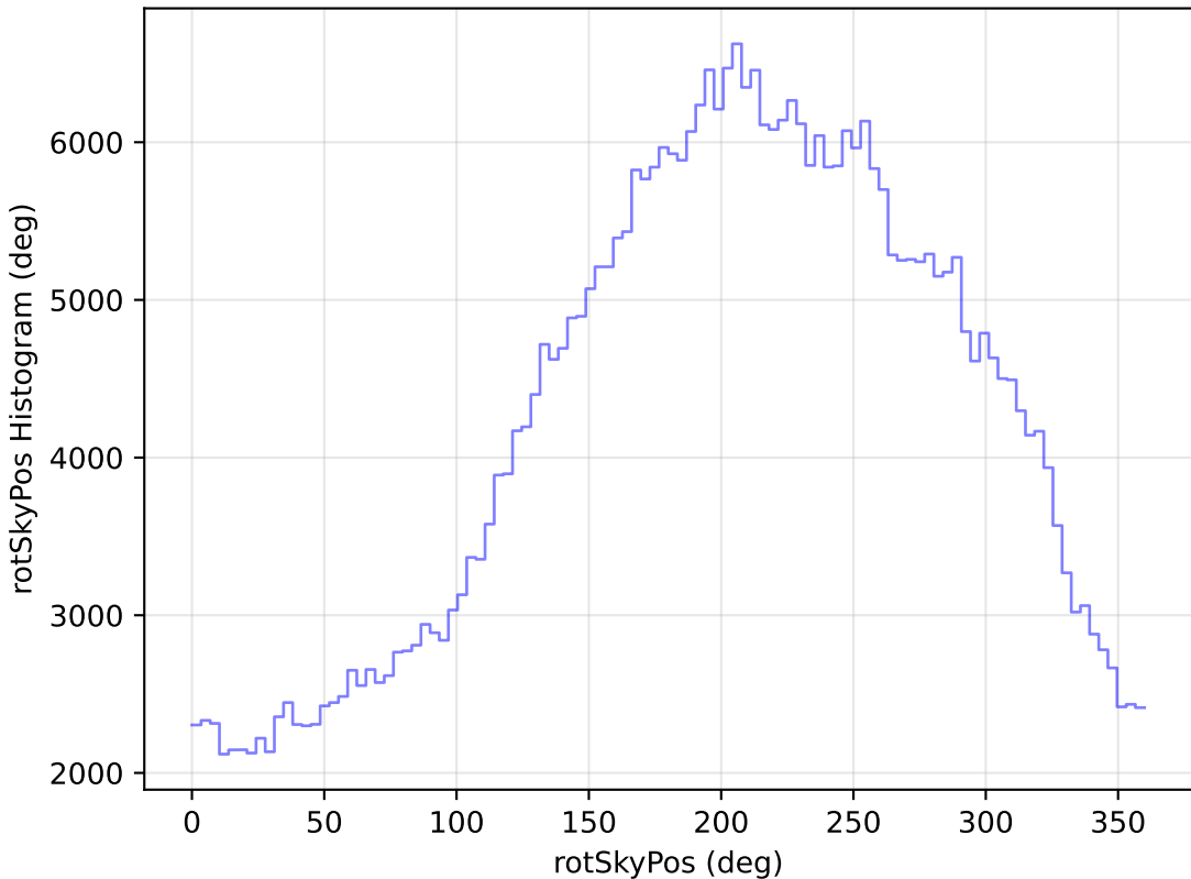
no_magell_roll_v3.4_10yrs All sky z band: rotSkyPos Histogram
