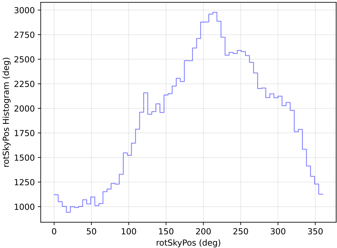
no_magell_roll_v3.4_10yrs All sky u band: rotSkyPos Histogram
