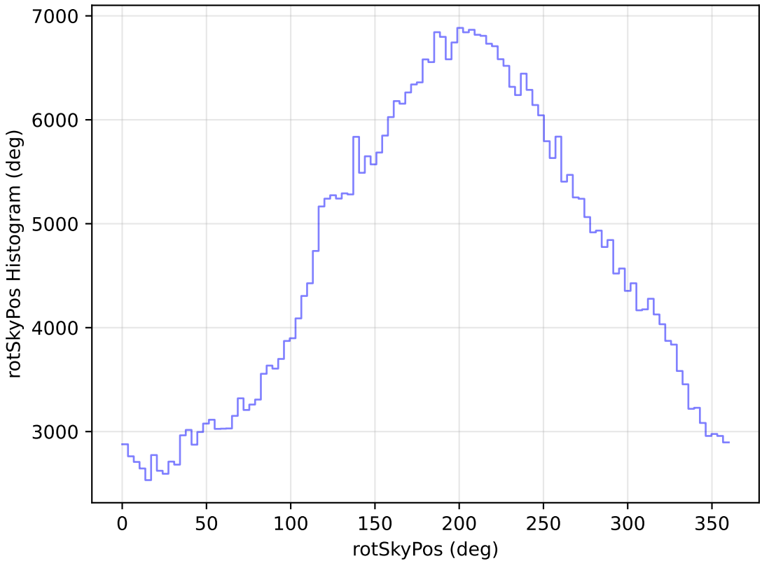
no_magell_roll_v3.4_10yrs All sky r band: rotSkyPos Histogram
